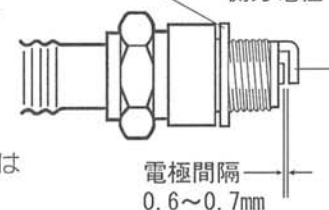
側方電極 (-)
