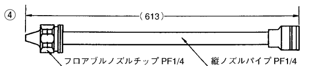
フロアブルノズルG1/4セット(パイプ付) G1/4
