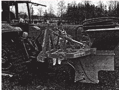
カットドレーナ
